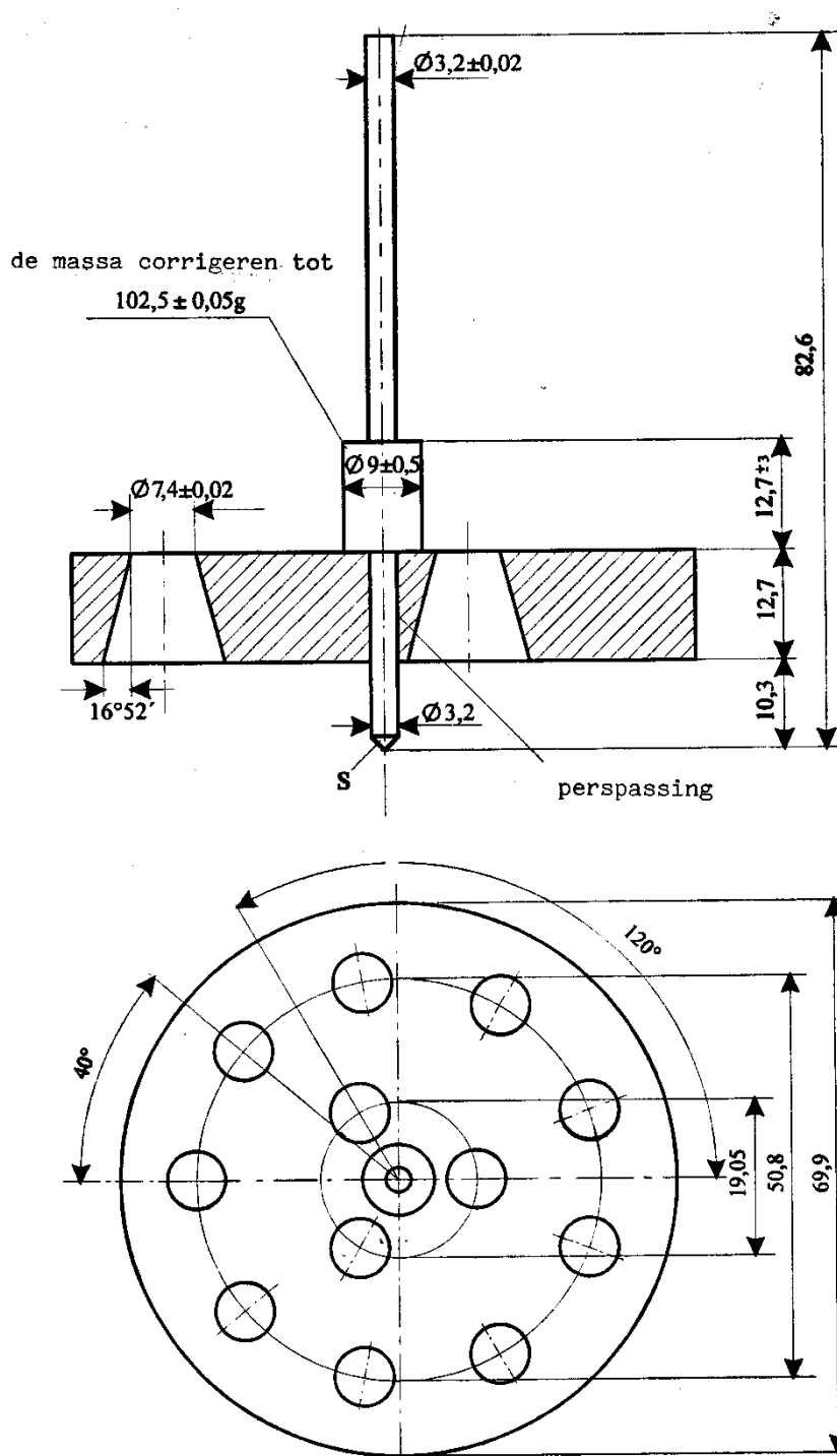
Figuur 1 Penetrometer
