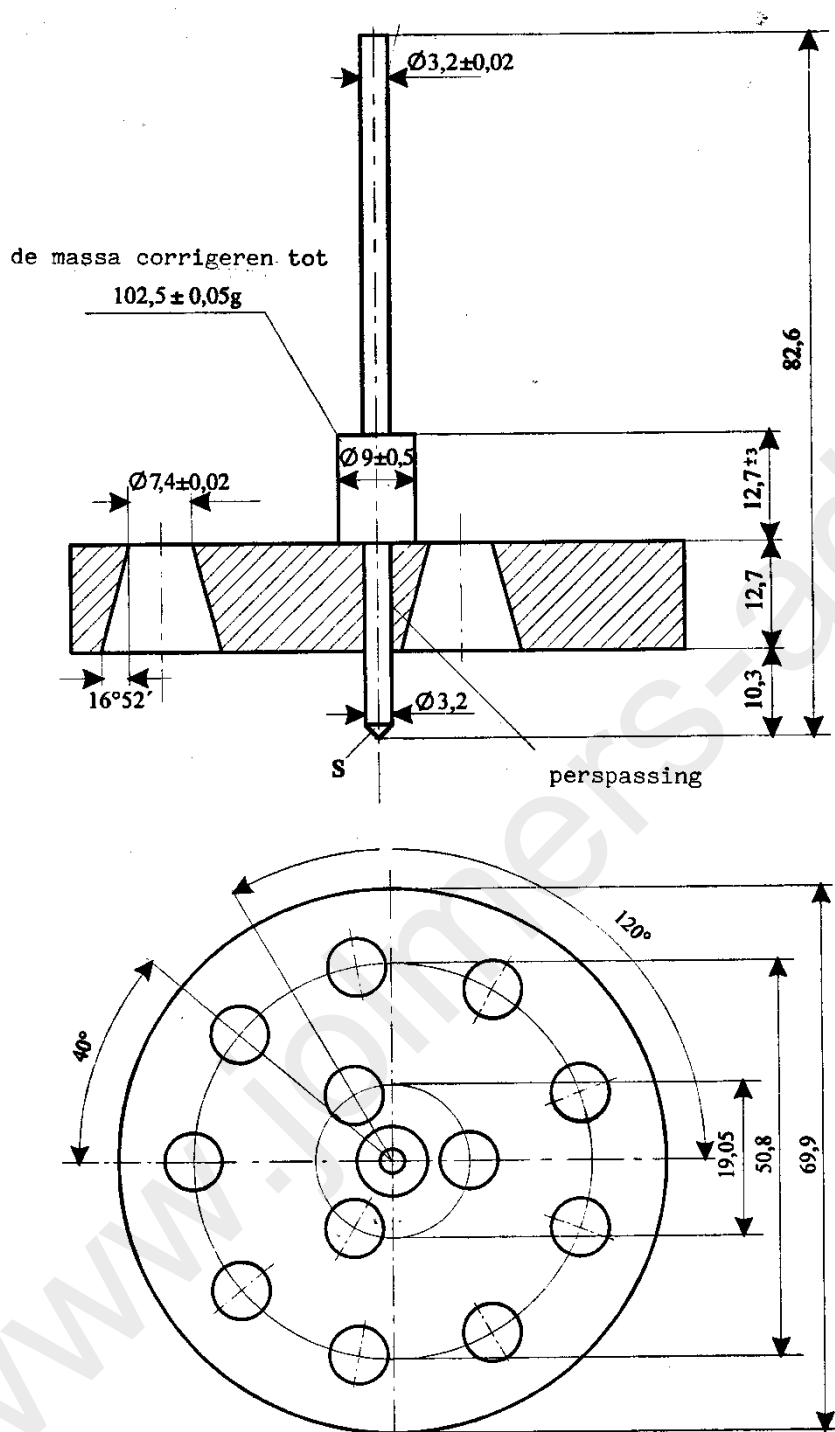
Figuur 1 Penetrometer
